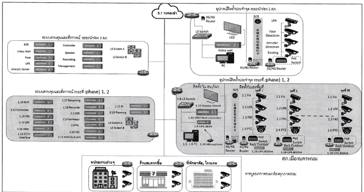
แผนผังภาพรวมการเชื่อมโยงระบบในภาพรวมโครงการ (System Diagram)
