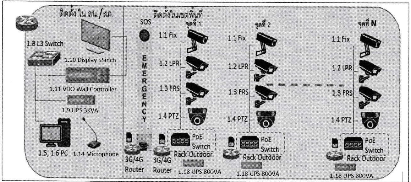
การออกแบบระบบอุปกรณ์ประจำสถานีตำรวจและพื้นที่รับผิดชอบ (Police Station Diagram)
